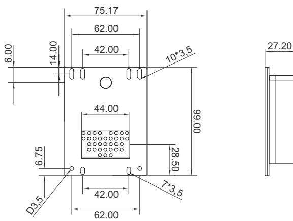
Lautsprecher ELA-100
