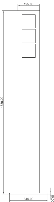
ELCOM.MODESTA Standssäule SMT 3/1
