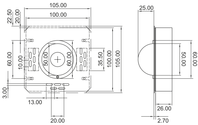
Kamera BTC-500
