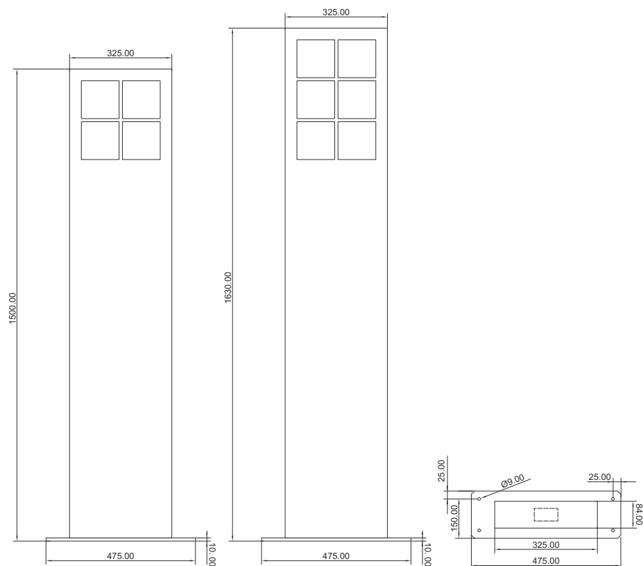
ELCOM.MODESTA Standssäule SMT 4-6/2
