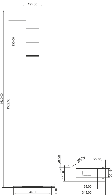
ELCOM.MODESTA Standssäule SMT 4/1
