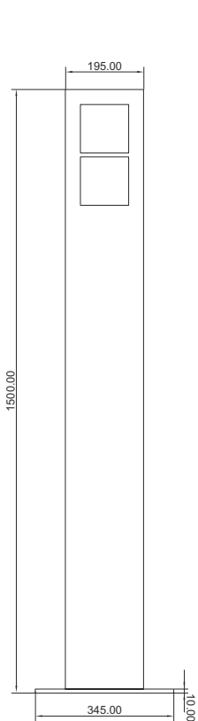
ELCOM.MODESTA Standssäule SMT 2/1
