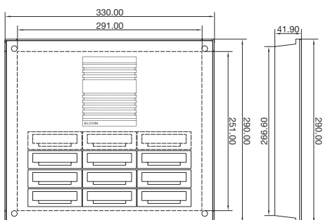
ELCOM.STABILA Aufputz 9- und 12-Ruftaster
